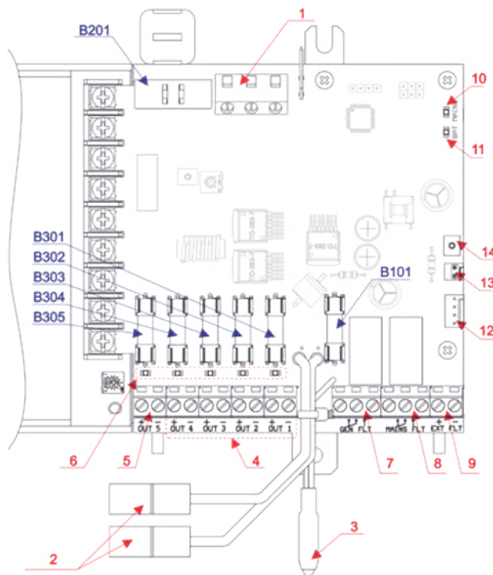
Fig. 4: Komponentplacering i strömförsörjningsmodul ZSPM-200
