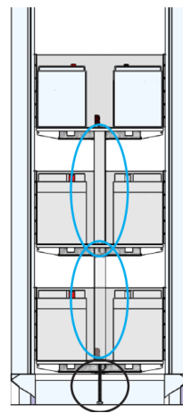
Figur 2. Golvstöd skall monteras på bägge storlekarna av batterihyllor.
