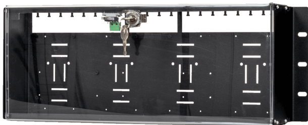
Plåtkapsling för 19" rack eller montering direkt på vägg, levereras med sabotagekontakt. 19 rack DIN module holder*
