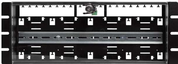
Plåtkapsling med DIN-skene för 19" rack eller montering direkt på vägg, levereras med sabotagekontakt.
